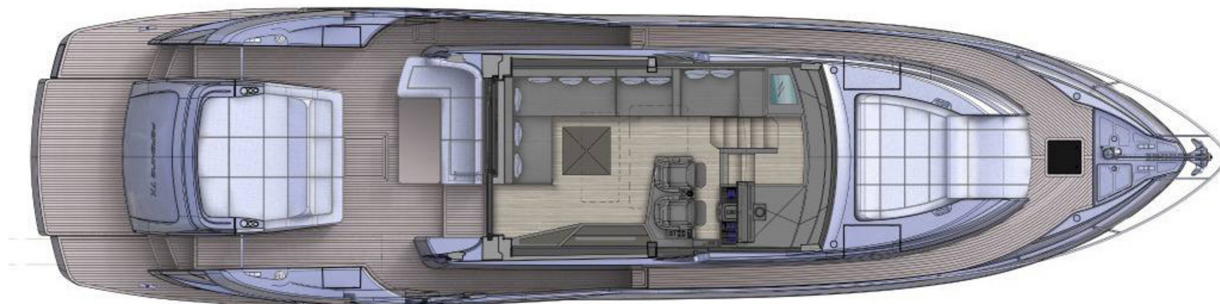
Планировка главной палубы
